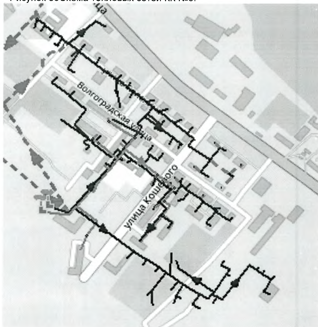
Рисунок 65 Схема тепловых сетей КК №6.
