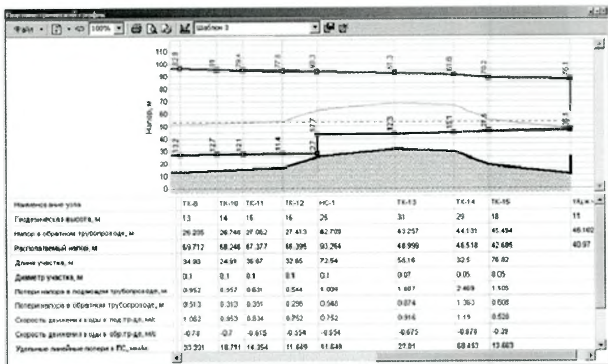
Рисунок 25. Пьезометрический график
