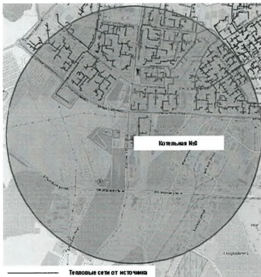
Рисунок 52 Радиус эффективного теплоснабжения котельной по улице Р.Фахретдина ООО Альтехносервис
