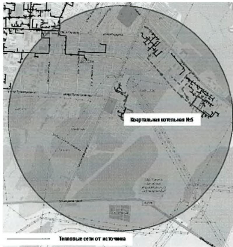
Рисунок 33 Радиус эффективного теплоснабжения квартальной котельной №5 АО АПТС
