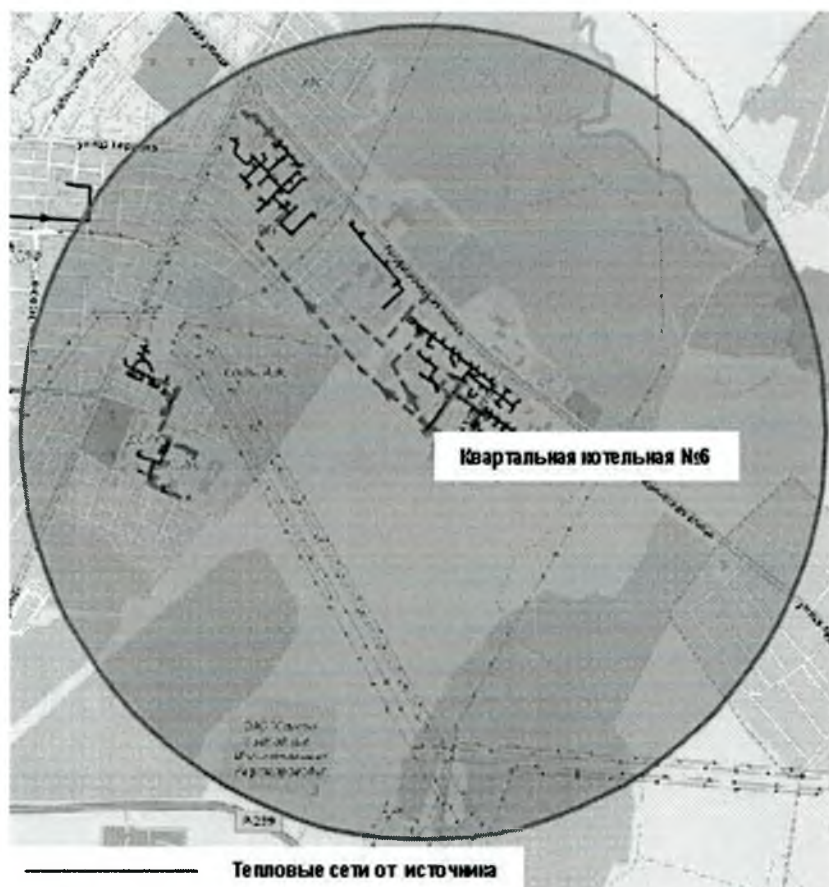
Рисунок 34 Радиус эффективного теплоснабжения квартальной котельной №6 АО АПТС
