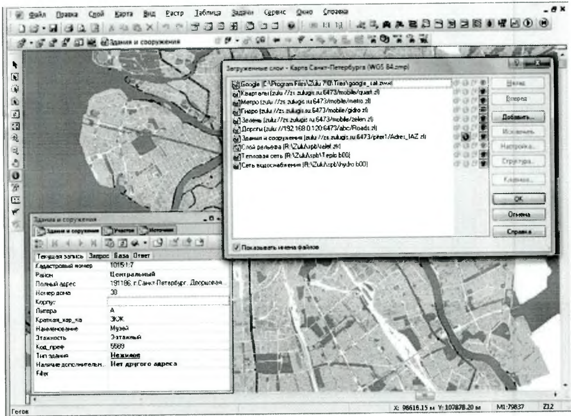
Рисунок 9. Векторные данные
