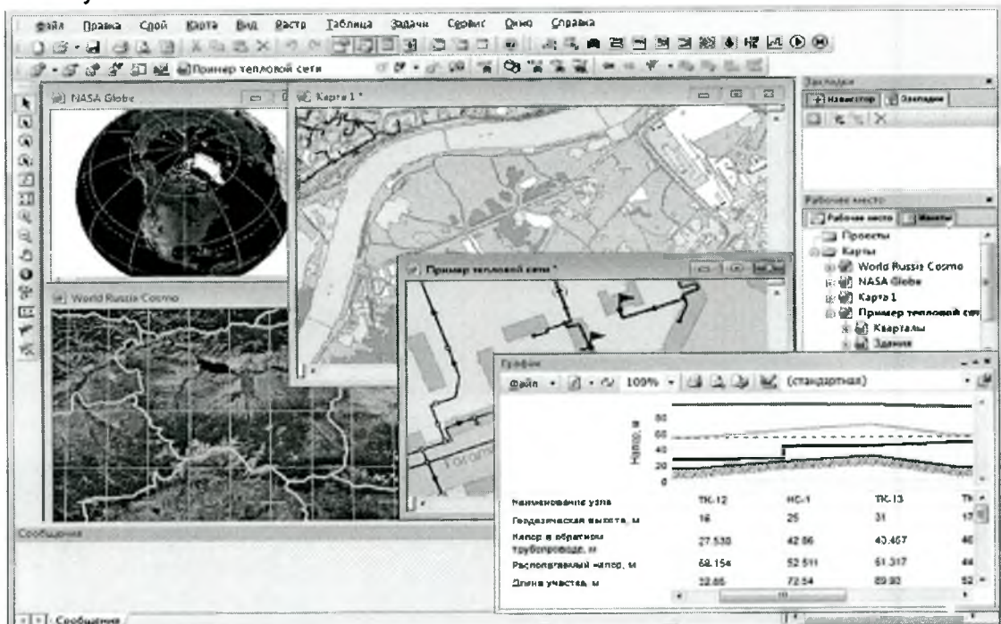
Рисунок 7. ГИС Zulu
